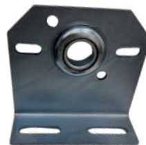
SOPORTE CENTRAL INDUSTRIAL ERREKA REF: SCI-CR AJUSTABLE CON RODAMIENTO Y REVESTIMIENTO DE ZING DE 3,0MM DE ESPESOR
